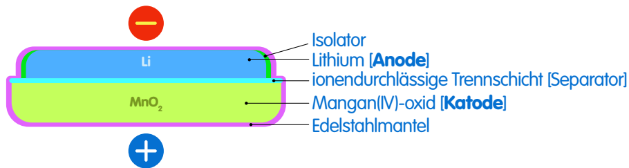
Lithium-Mangandioxid-Knopfzelle eqjooki.de
