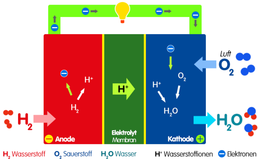
PEM-Brennstoffzelle [Prinzip]
